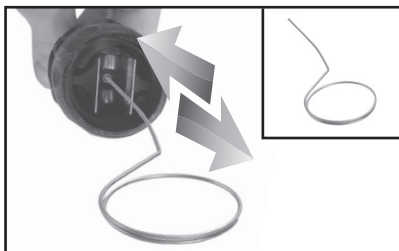
Fűvóka tisztító tű, 13. ábra
